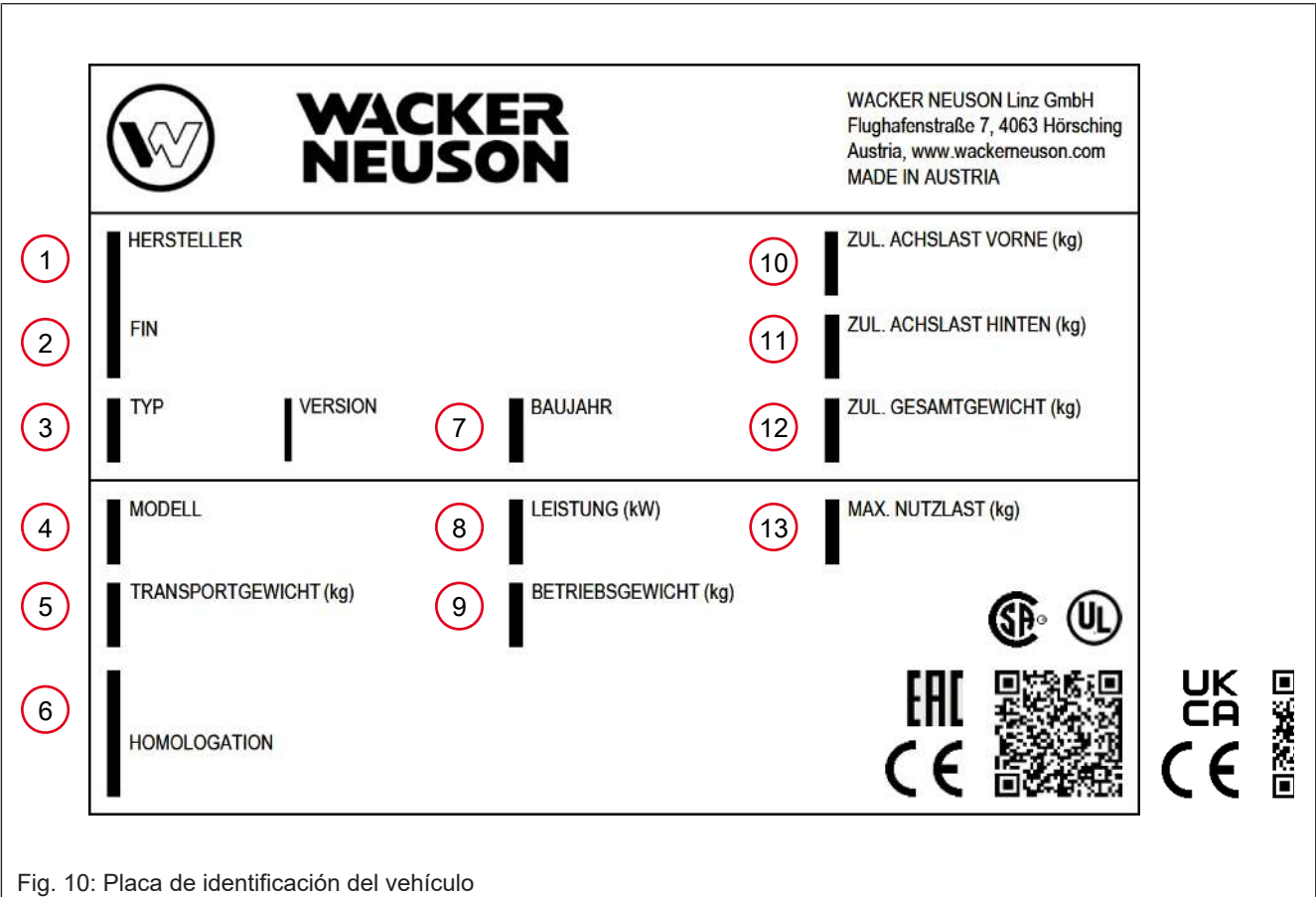
Fig. 10: Placa de identificación del vehículo
