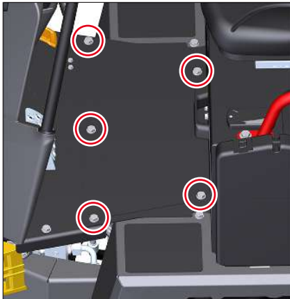
Fig. 101: Chapa de piso
