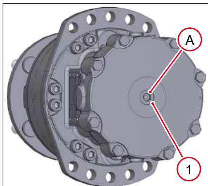
Fig. 107: Desactivar el freno de estacionamiento
