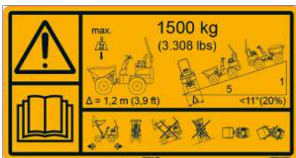
Fig. 17: Funcionamiento seguro
