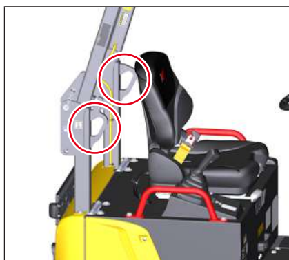
Fig. 114: Cáncamos de elevación barra antivuelco
