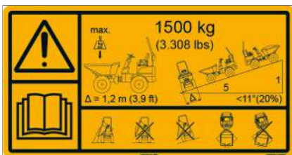
Fig. 16: Funcionamiento seguro
