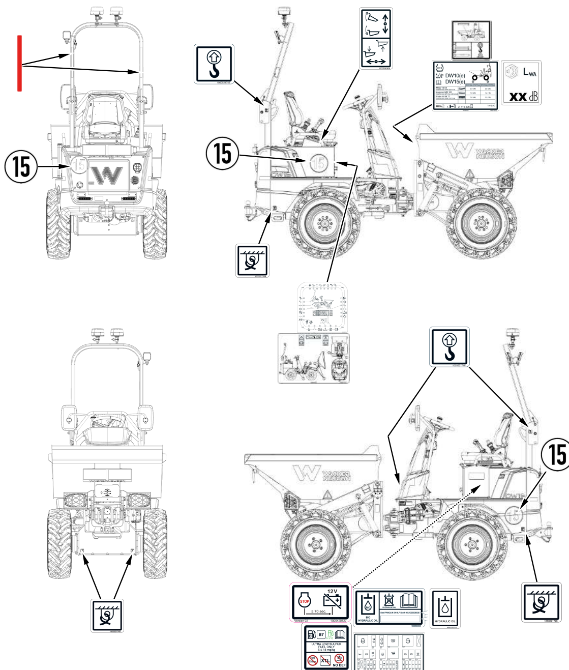
Fig. 24: Vista general de los adhesivos de indicaciones
