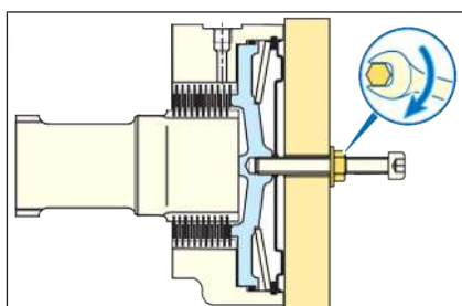
Fig. 108: Desactivar el freno de estacionamiento
