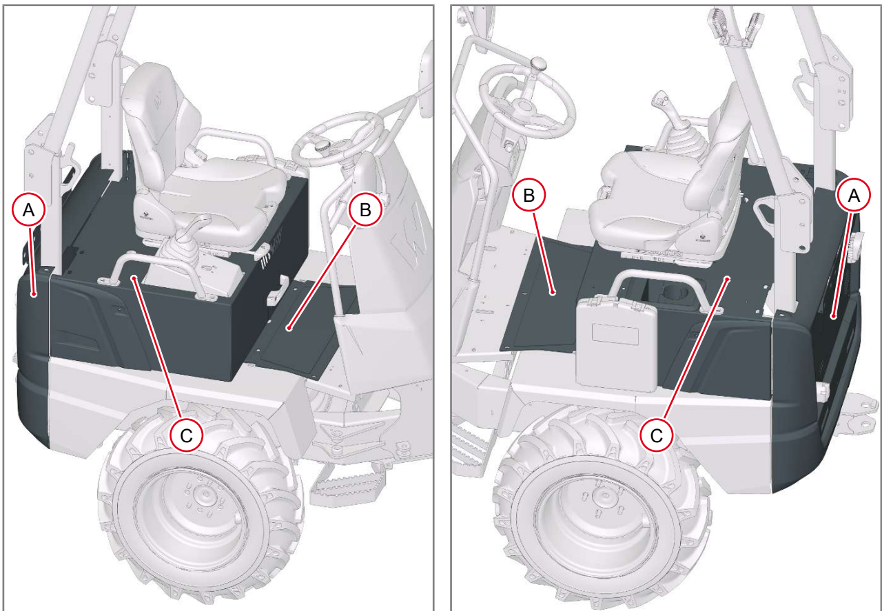
Fig. 120: Accesos de mantenimiento
