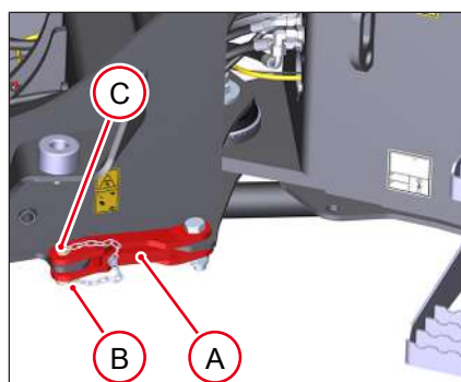
Fig. 110: Bloqueo articulado desmontado
