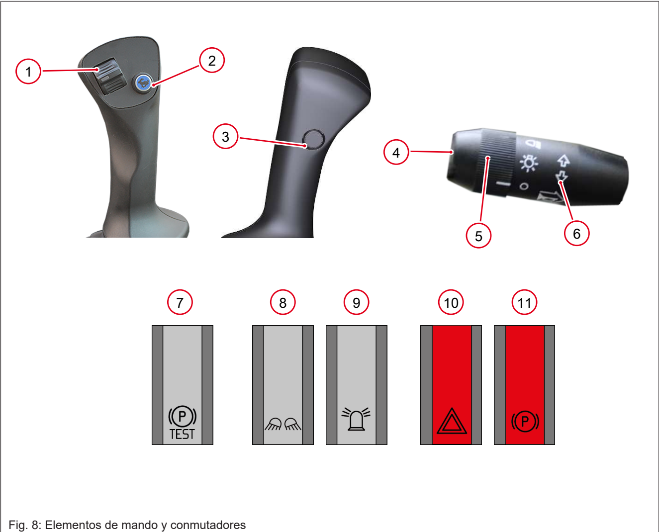
Fig. 8: Elementos de mando y conmutadores
