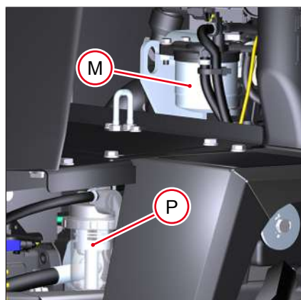
Fig. 130: Filtro previo y principal de combustible
