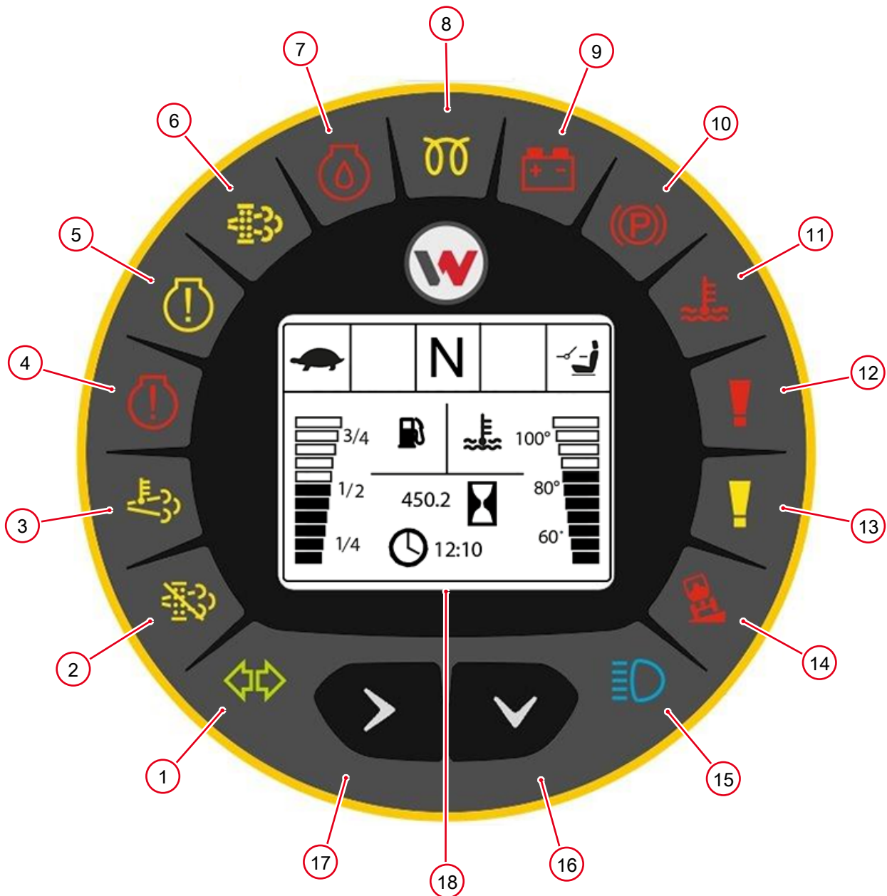
Fig. 52: Luces de control
