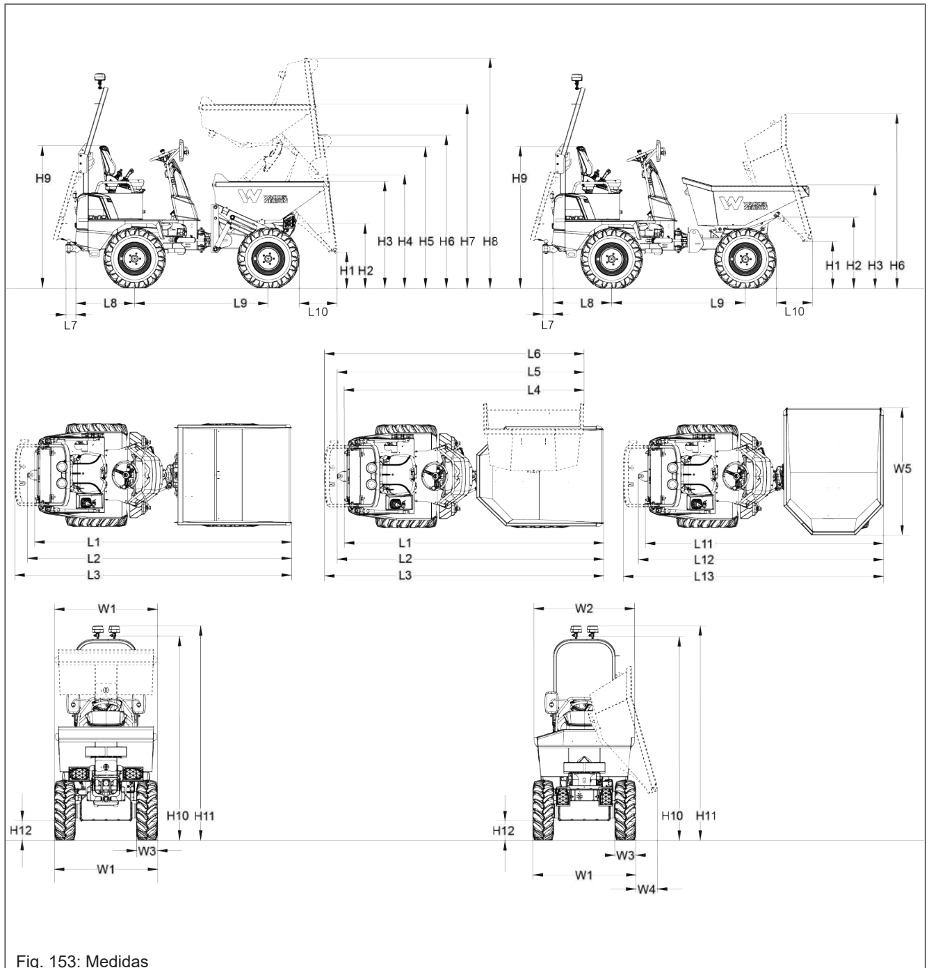
Fig. 153: Medidas
