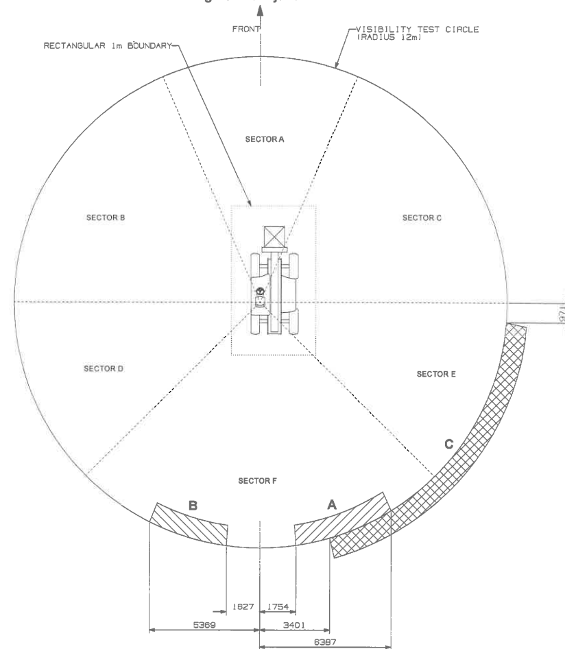
Figura 218. Ajuste del retrovisor
