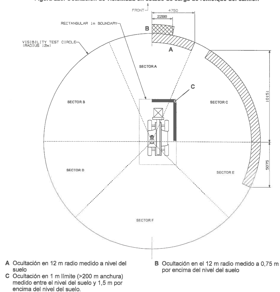
Figura 220. Ocultación de visibilidad en estado de carga de remolque del camión
