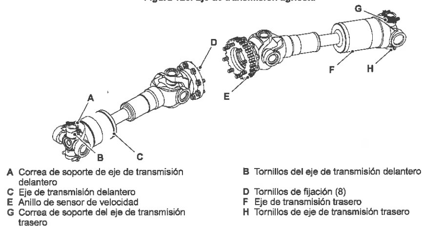
Figura 128. Eje de transmisión agrícola
