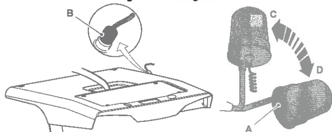
Figura 41. Abisagrado
