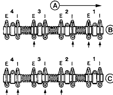
A—Parte delantera del motor E—Válvula de escape B—Pistón No. 1 en PMS de la carrera de compresión I— Válvula de admisión C—Pistón número 4 en PMS de la carrera de compresión
