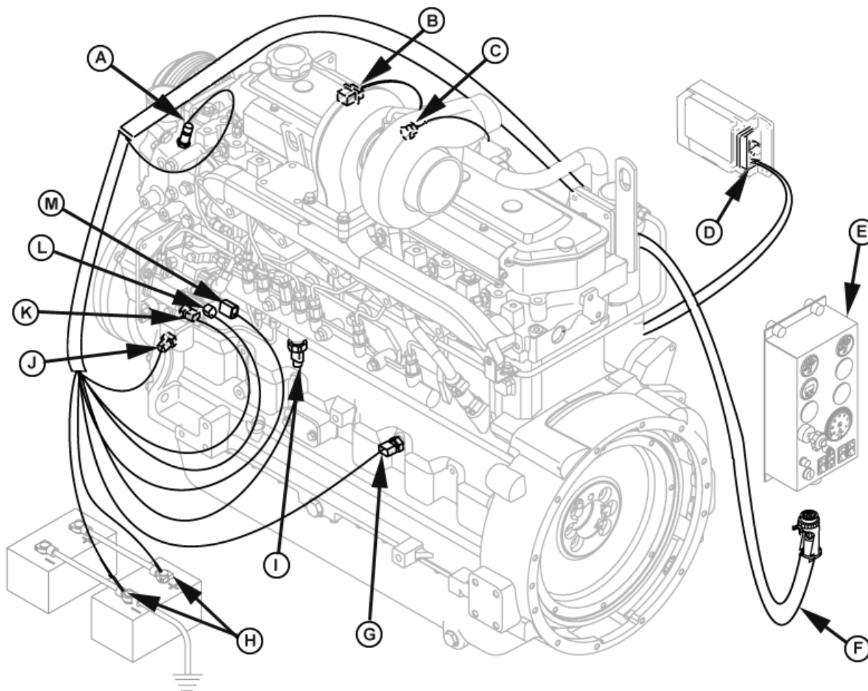
Motor 6068HFU72
