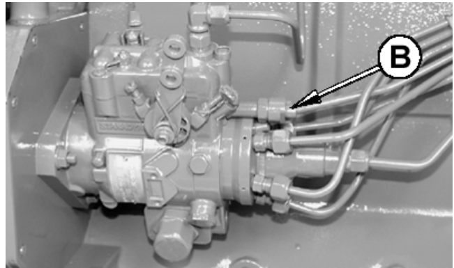
B—Tornillo de ajuste del regulador de variación de velocidad
