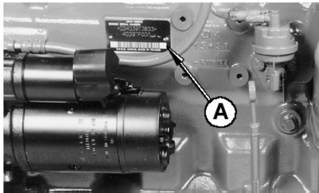
Motores 3029 y 4039
