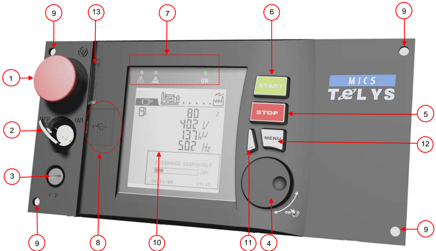
Figura 6.4 : Presentación de la parte delantera
