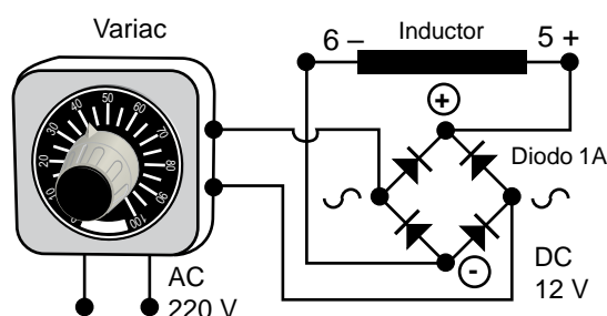
Montaje B
