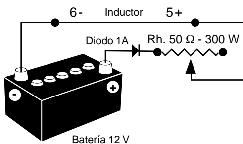
Montaje A
