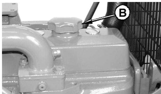
Motores 4045 y 6068
