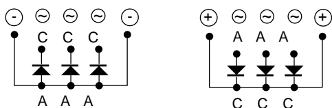
Puente de diodos LSA 43.2 / 44.2
