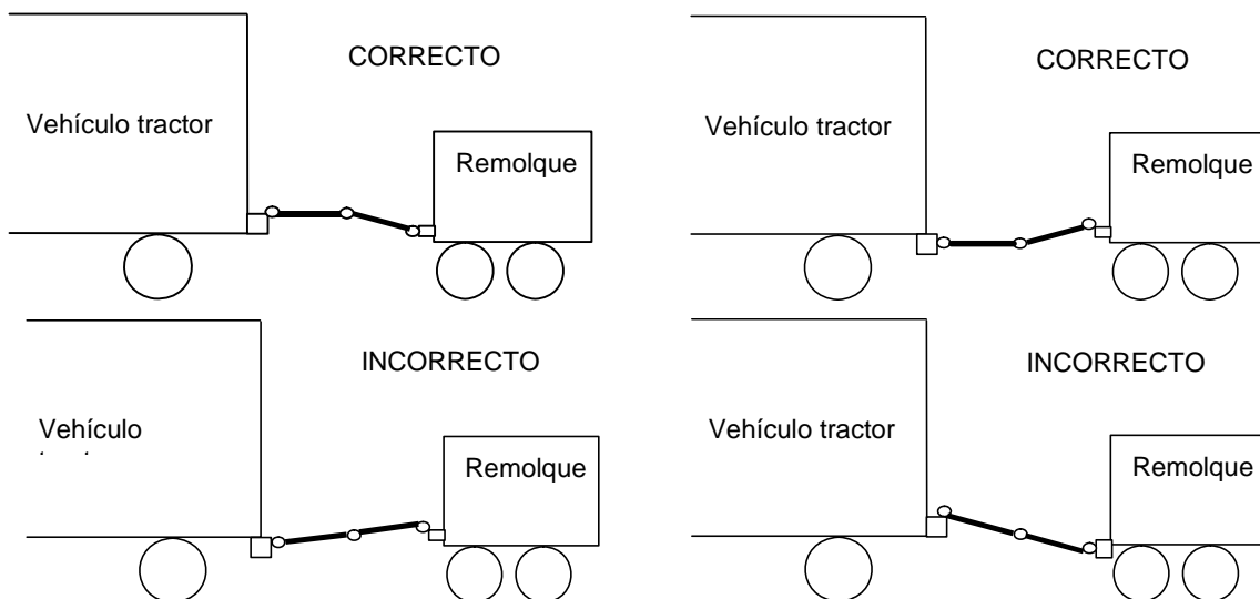
Figura 4.1 : Enganche de un remolque
