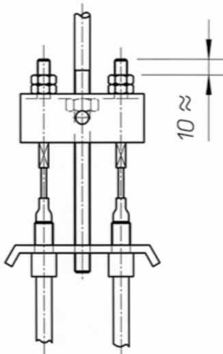
Figura 4.4- Montaje de la vigueta de elevación
