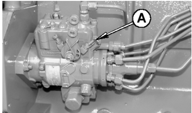
A—Tornillo ajuste régimen rápido
