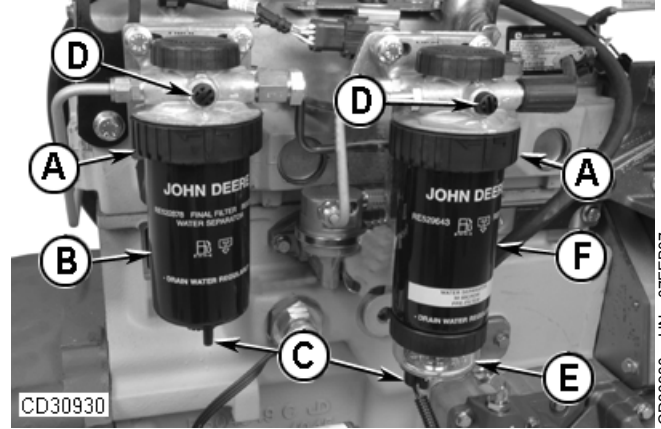
Combustible, filtros
