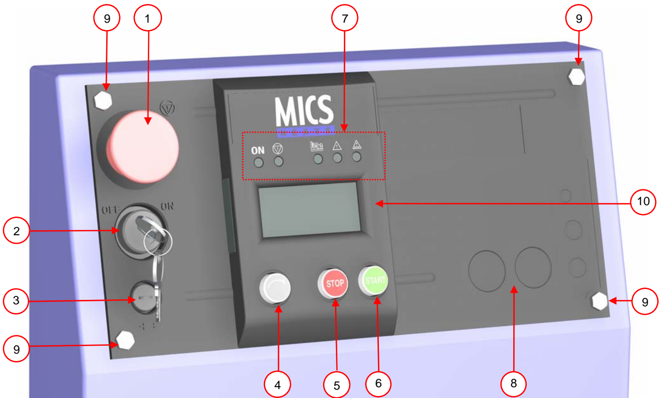
Figura 6.1 : Presentación de la parte delantera
