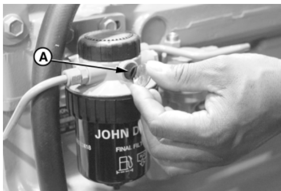
Tronillo de purga del filtro de combustible
