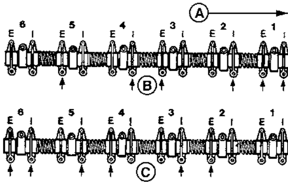
A—Parte delantera del motor E—Válvula de escape B—Pistón No. 1 en PMS de la carrera de compresión I— Válvula de admisión C—Pistón número 4 en PMS de la carrera de compresión
