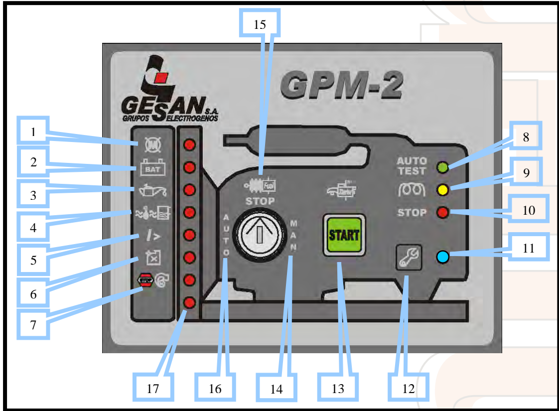
Imagen 10- Placa de Control GPM-2
