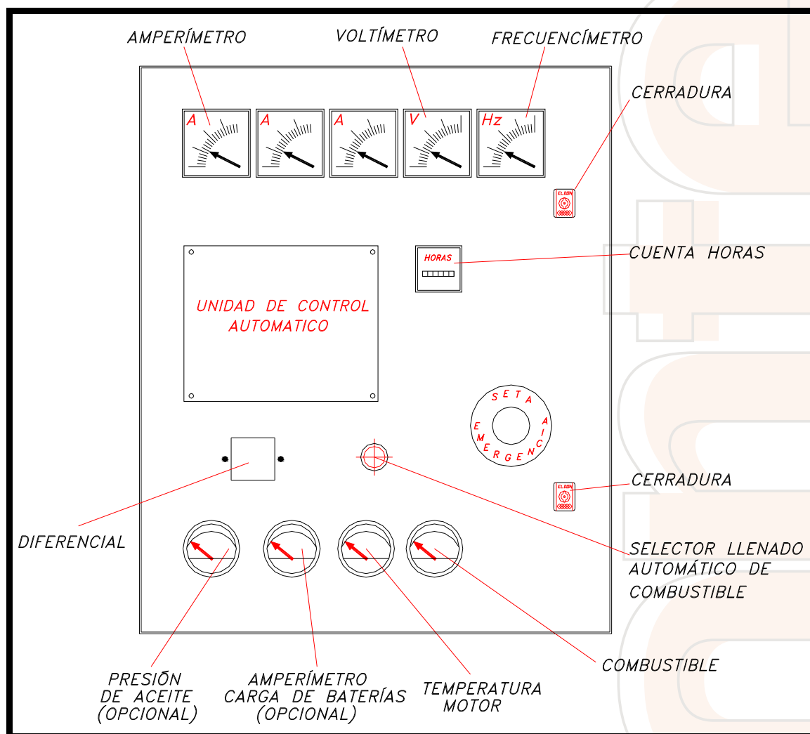
Imagen 4- Cuadro de Control genérico
