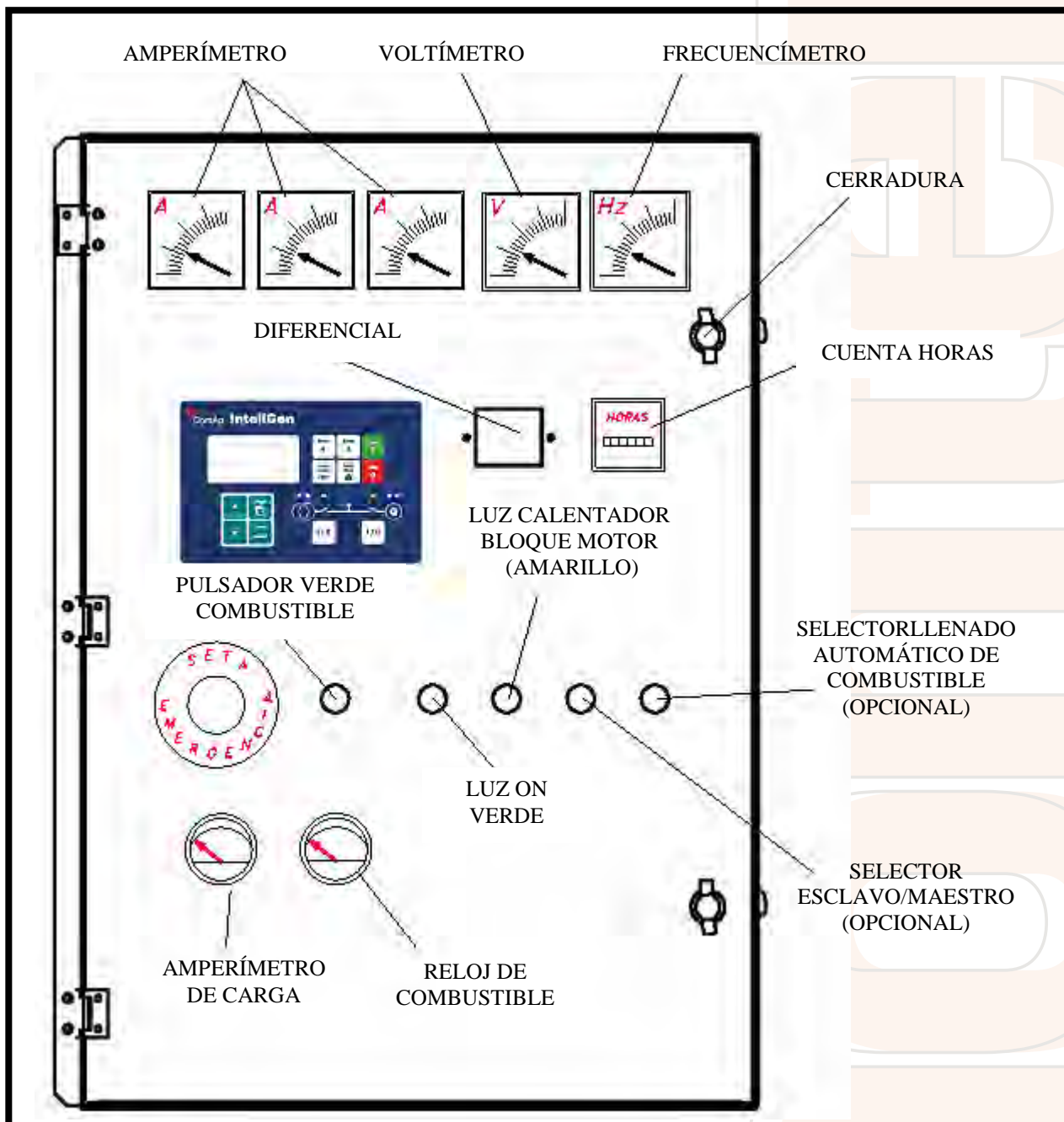
Imagen 7- Cuadro de Control de Placa de Control IntelGen
