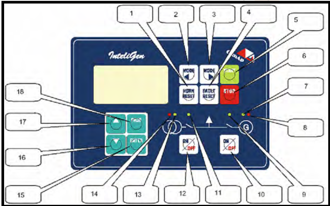
Imagen 14- Placa de Control IntelliGen
