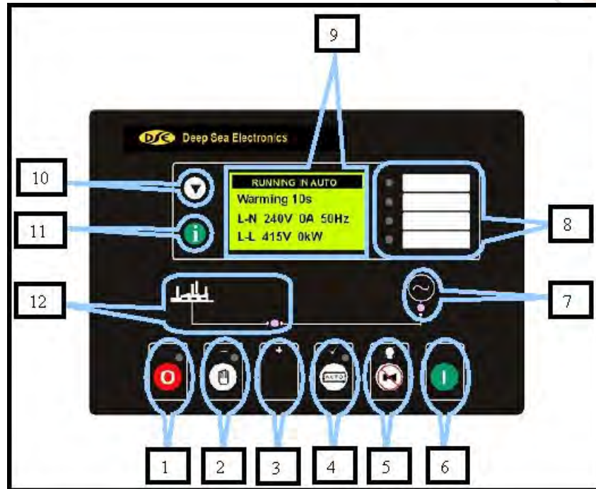
Imagen 13- Placa de Control DeepSea 5310
