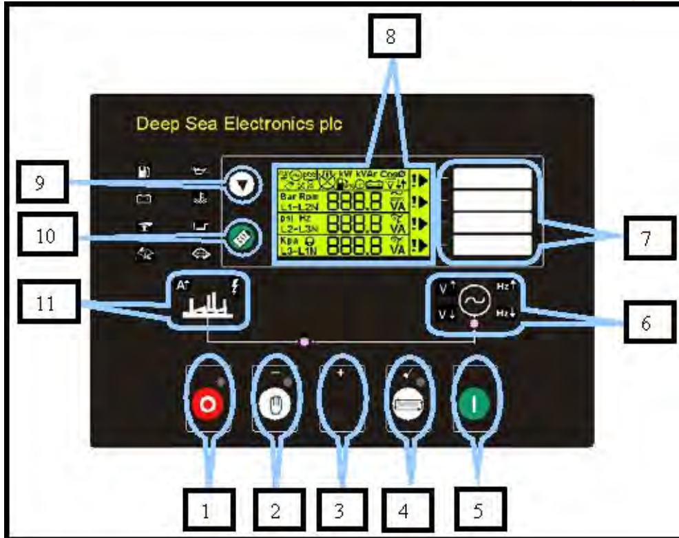
Imagen 11- Placa de Control DeepSea 5210
