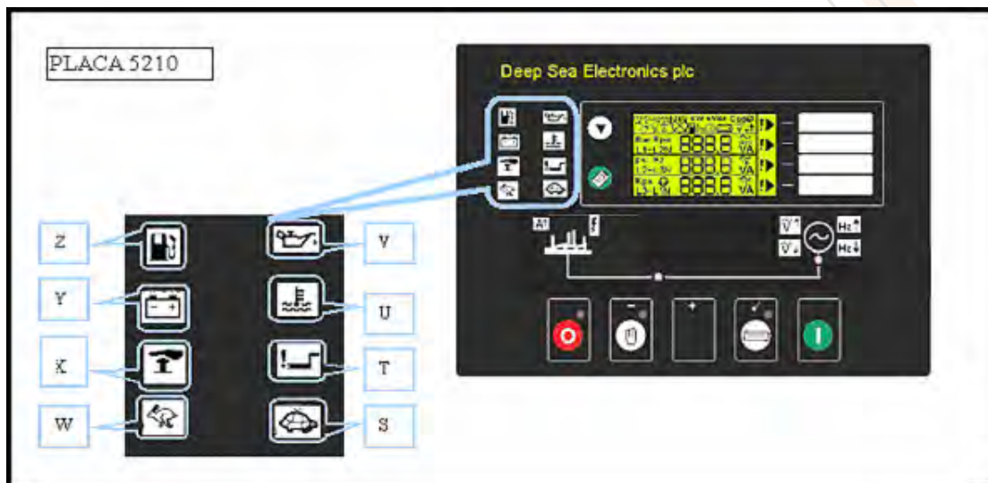
Imagen 12- Placa de Control DeepSea 5210
