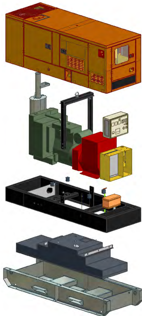
Imagen 2- Despiece de Imagen 1
