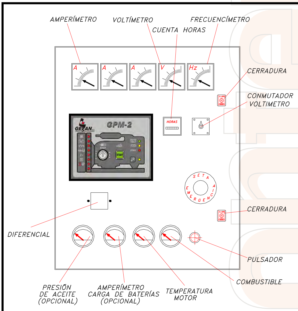
Imagen 5 - Cuadro de Control de Placa de Control GPM-2
